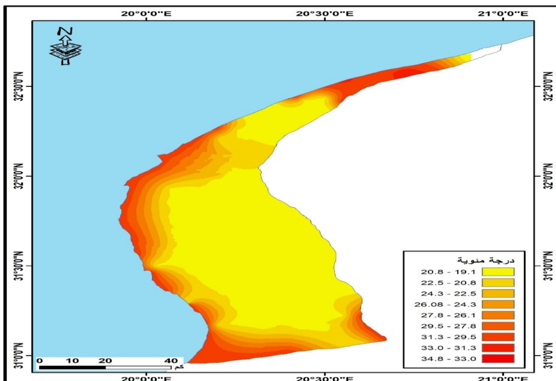
خريطة (2): خطوط الحرارة المتساوية بسهل بنغازي.
