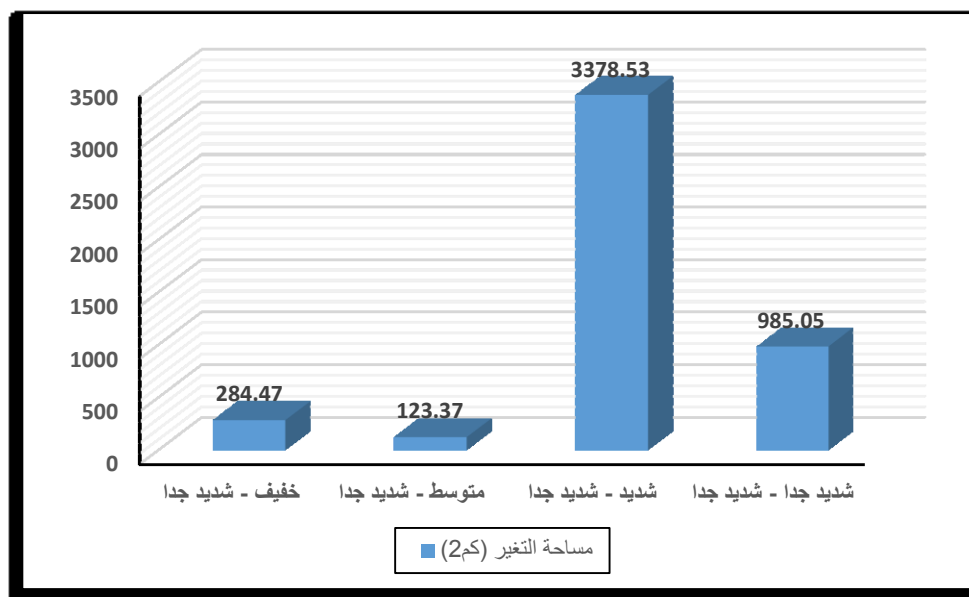
شكل(3): مساحات التغير بالتصحر (1984 - 2019).
