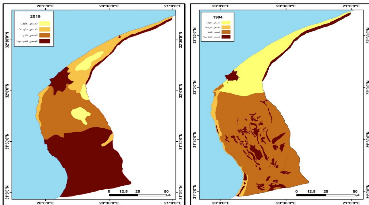
خريطة (5) : درجات تصحر سهل بنغازي لعامي 1984، 2019.
