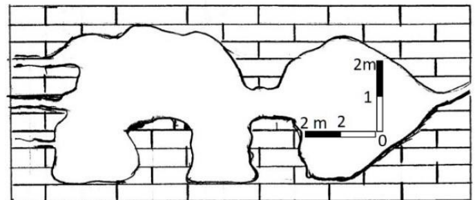
Fig. 24. Cross Section A-A'
