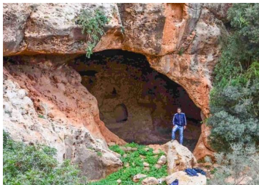
Fig. 25. Entrance of Wadi Belgares Cave
