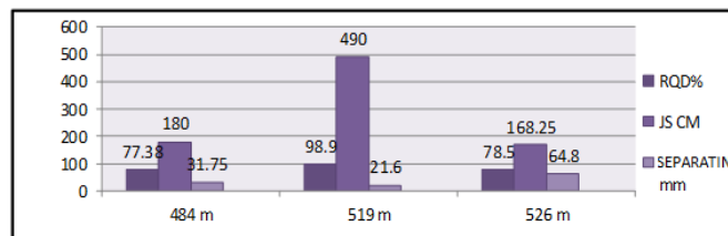
شكل 6. العلاقة بين الارتفاع والخواص الهندسية في الموقع (L-Ja-17).
