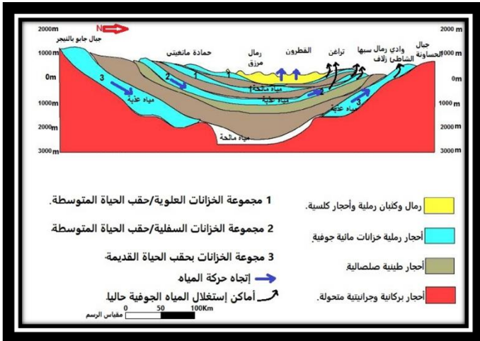
شكل 3. قطاع هيدرولوجي يبين الخزانات المائية بحوض مرزق (Pallas, 1980)
